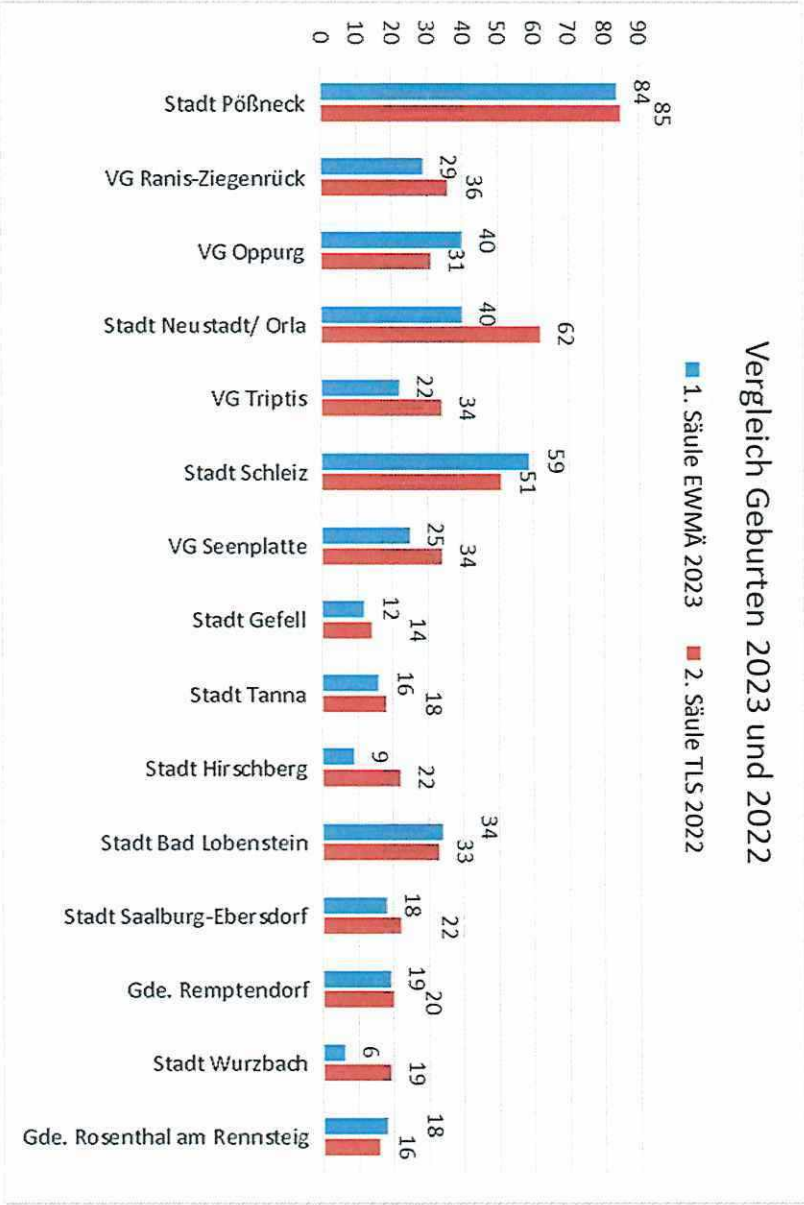
Abbildung 2: Vergleich Geburten 2022 - 2023
